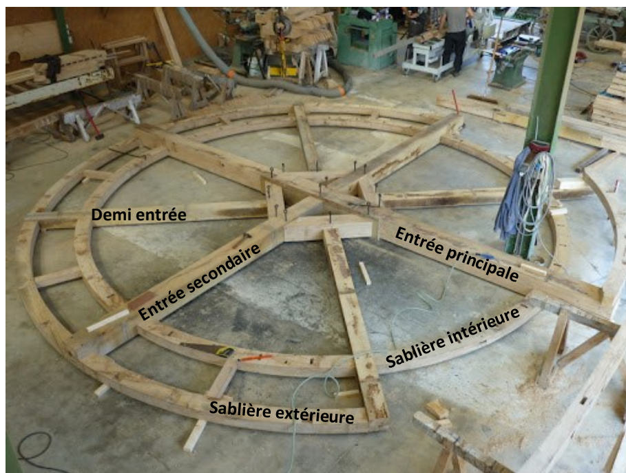
Deux exemples d'assemblage de la partie horizontale de la future charpente
