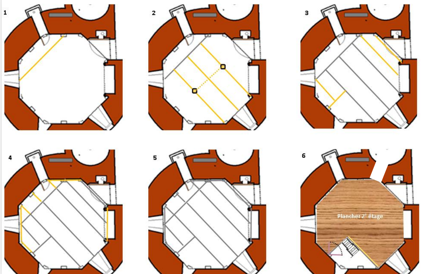
Schématisation du solivage du plancher du 2° étage de la tour Jourdain
